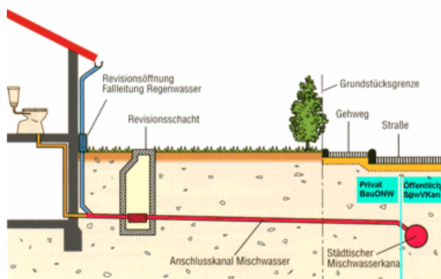
Kanäle und Leitungen im Mischsystem
